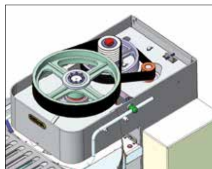
Trasmissione Heavy Duty a doppio invio Heavy Duty double transmission
